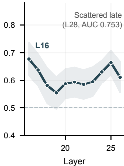
Llama-3.1-8B
