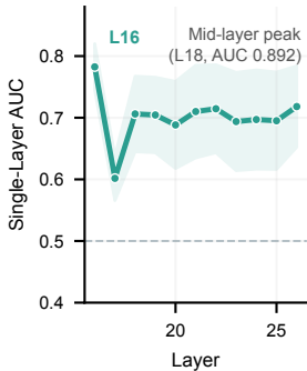
Mistral-7B-v0.3
