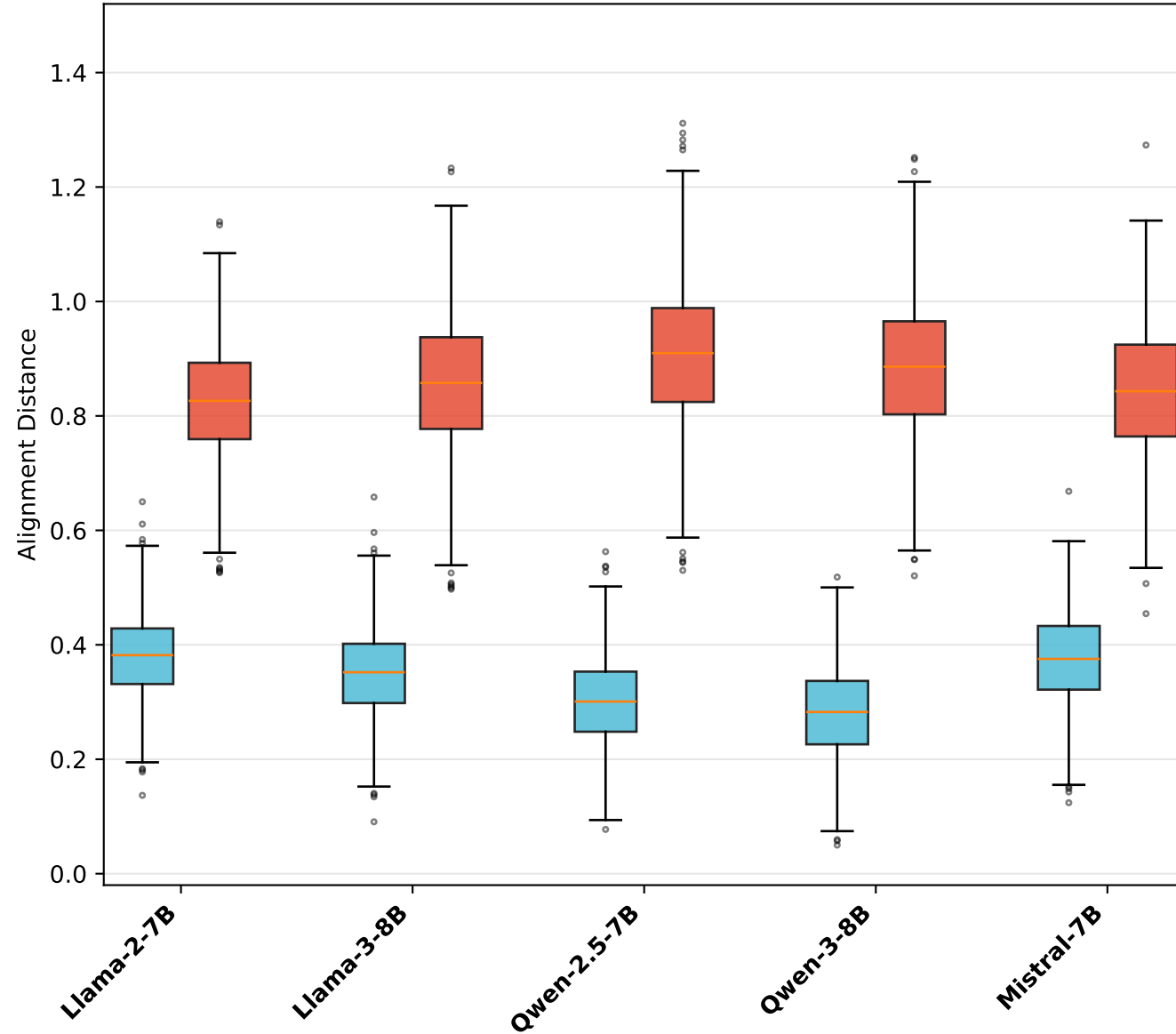
PubMedQA
