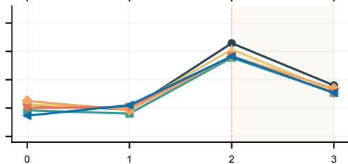
Llama-3-8B
