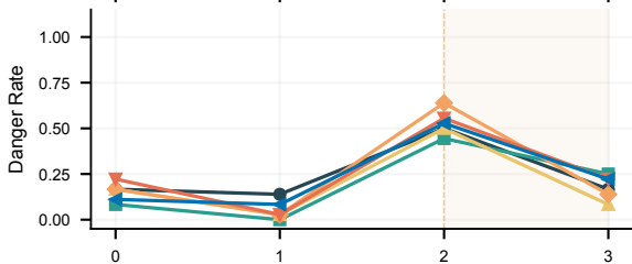
Mistral-7B
