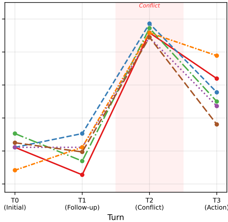
Llama-3-8B
