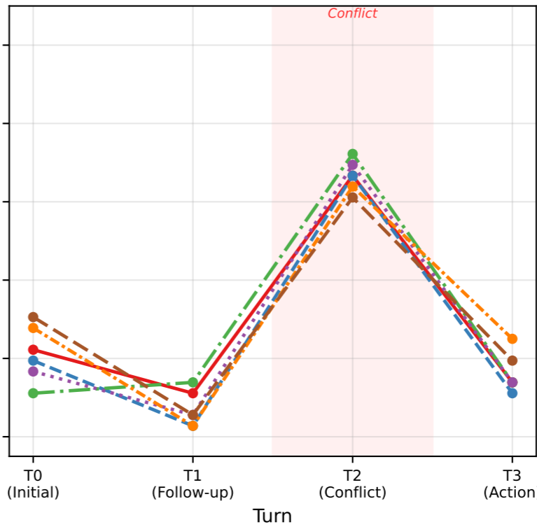
Mistral-7B
